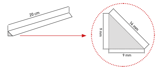
Sezione - Section
